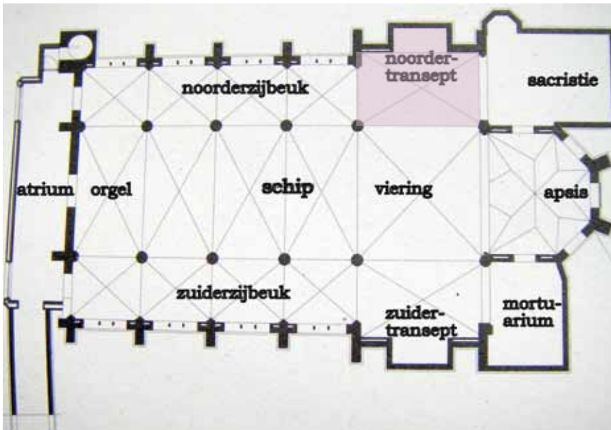
Plattegrond kapel Moederhuis DMJ. Met viering wordt hier bedoeld een bouwkundige viering, zijnde de ruimte tussen vier zuilen onder de dakruiter (klokkentorentje).
